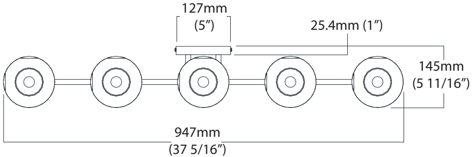
Top View / Vue de Dessus
