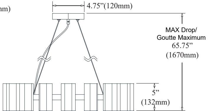
Front view Vue de face
