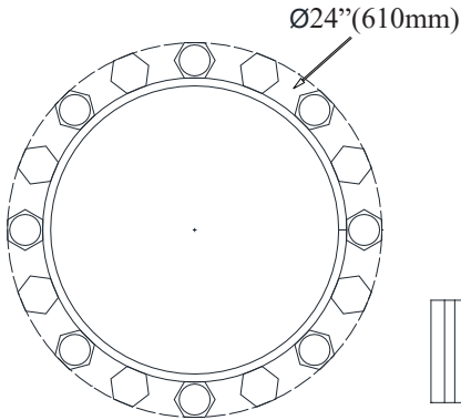
Top view Vue de dessus
